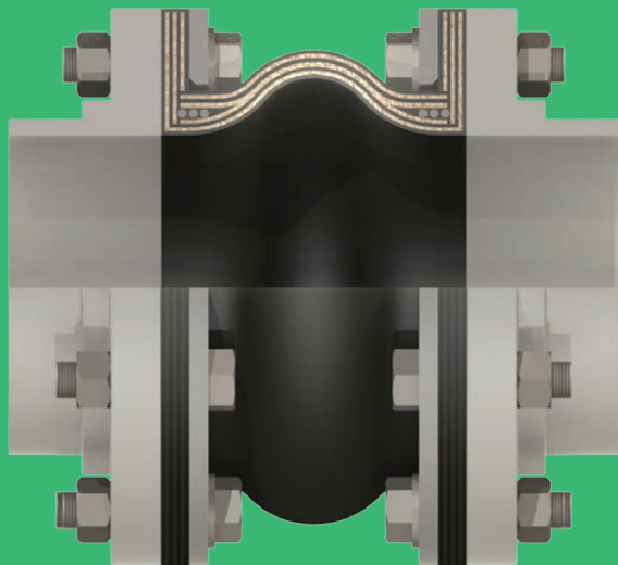
Style 261R
